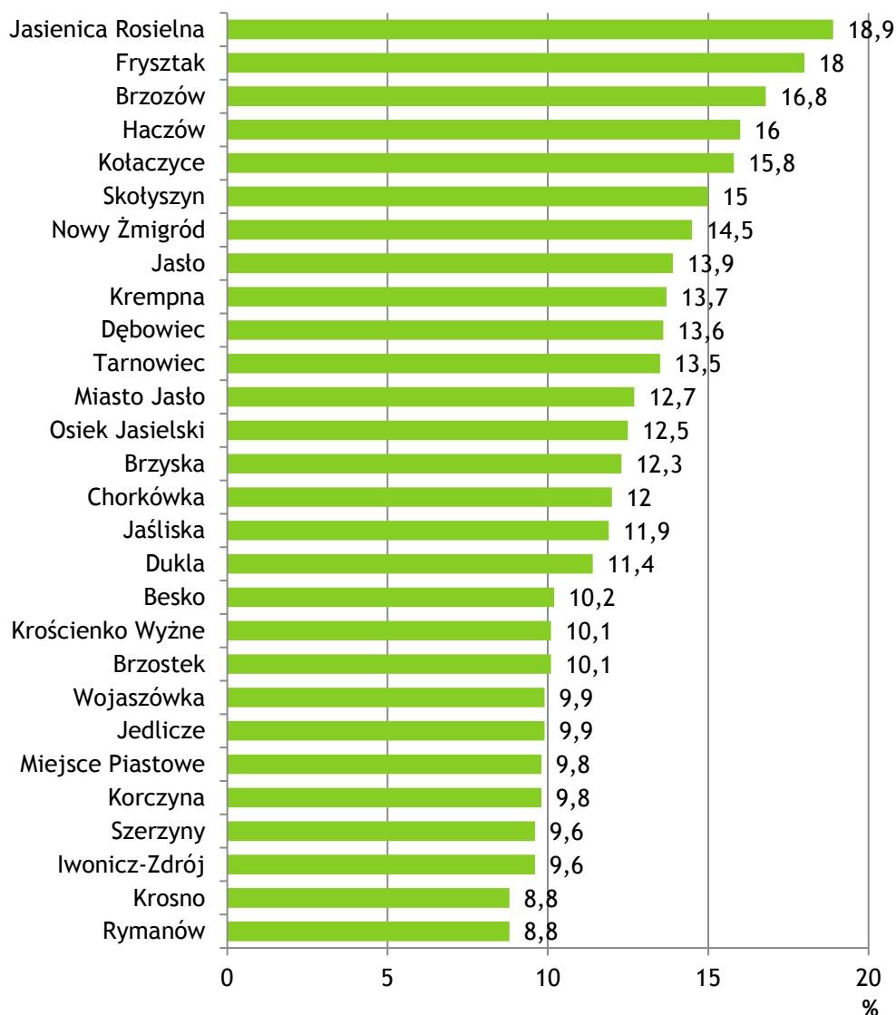
Wykres 7. Udział zarejestrowanych bezrobotnych w liczbie ludności w wieku produkcyjnym w roku 2013
